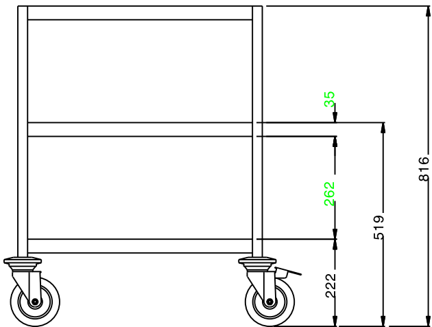
Zij aanzicht
